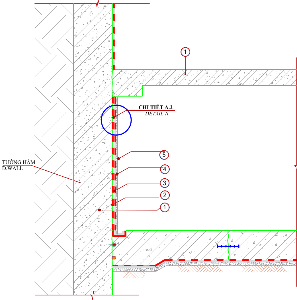
BIỆN PHÁP THI CÔNG CHỐNG THẤM TƯỜNG VÂY + ĐÁY SÀN HẦM WATERPROOFING M.S FOR D.WALL - BASEMENT SLAB
