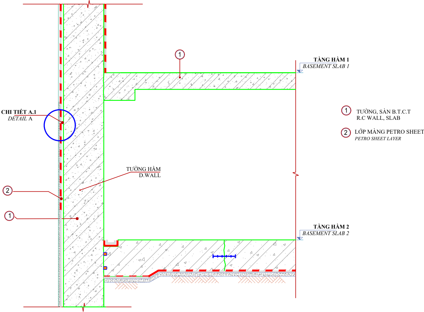
BIỆN PHÁP THI CÔNG CHỐNG THẤM TƯỜNG VÂY + ĐÁY SÀN HẦM WATERPROOFING M.S FOR D.WALL - BASEMENT SLAB
