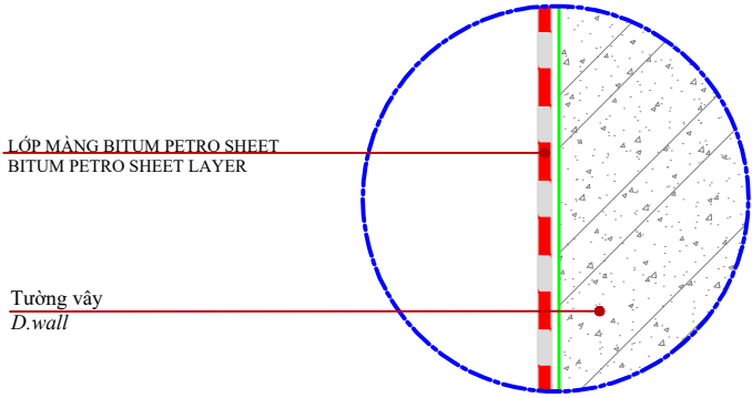
CHI TIẾT A DETAIL A
