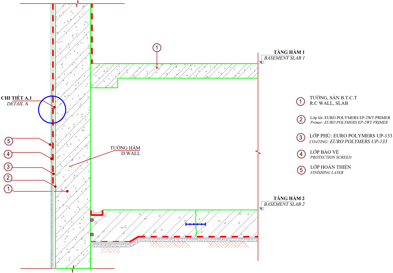
BIỆN PHÁP THI CÔNG CHỐNG THẤM TƯỜNG VÂY + ĐÁY SÀN HẦM WATERPROOFING M.S FOR D.WALL - BASEMENT SLAB
