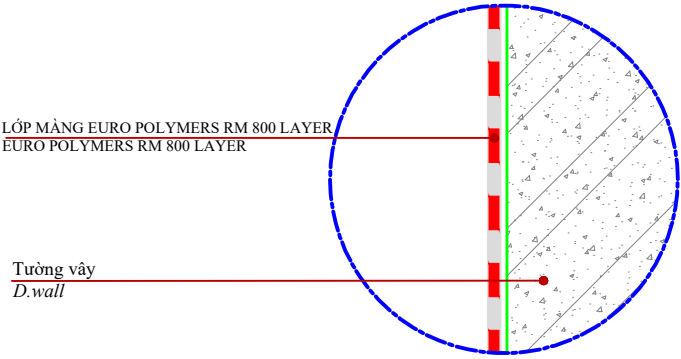
CHI TIẾT A DETAIL A
