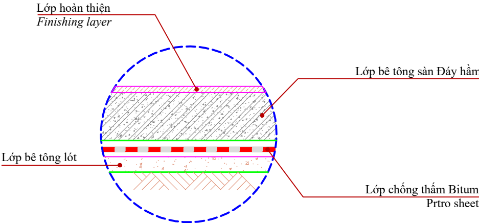
CHI TIẾT B DETAIL B
