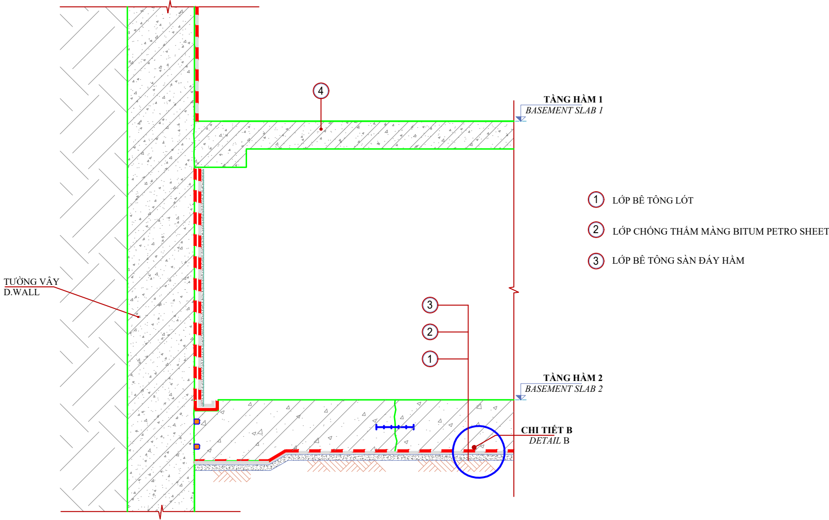
BIỆN PHÁP THI CÔNG CHỐNG THẤM TƯỜNG VÂY + ĐÁY SÀN HẦM WATERPROOFING M.S FOR D.WALL - BASEMENT SLAB
