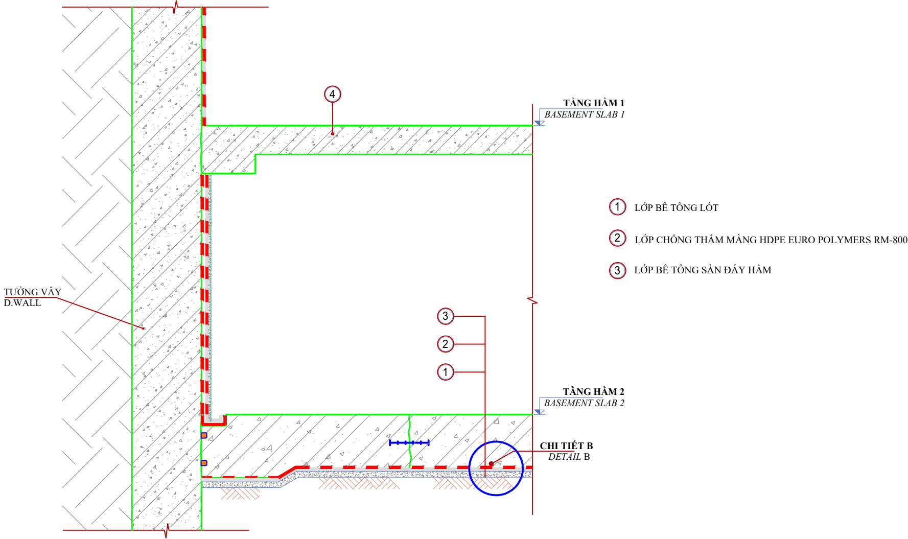
BIỆN PHÁP THI CÔNG CHỐNG THẤM TƯỜNG VÂY + ĐÁY SÀN HẦM WATERPROOFING M.S FOR D.WALL - BASEMENT SLAB
