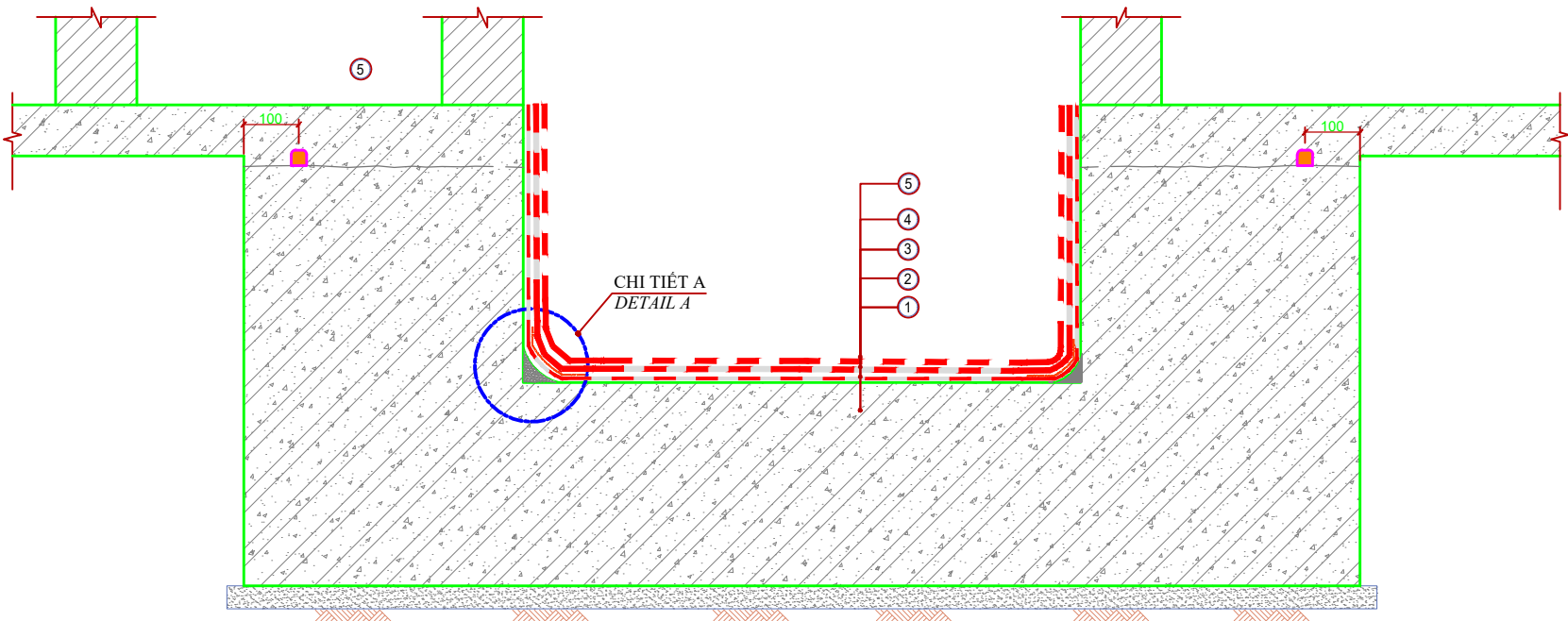
BIỆN PHÁP THI CÔNG CHỐNG THẤM HỒ THANG MÁY WATERPROOFING METHOD STATEMENT FOR LIFT PIT
