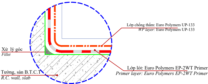
CHI TIẾT A DETAIL A
