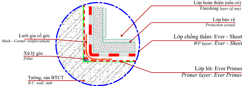
CHI TIẾT A DETAIL A
