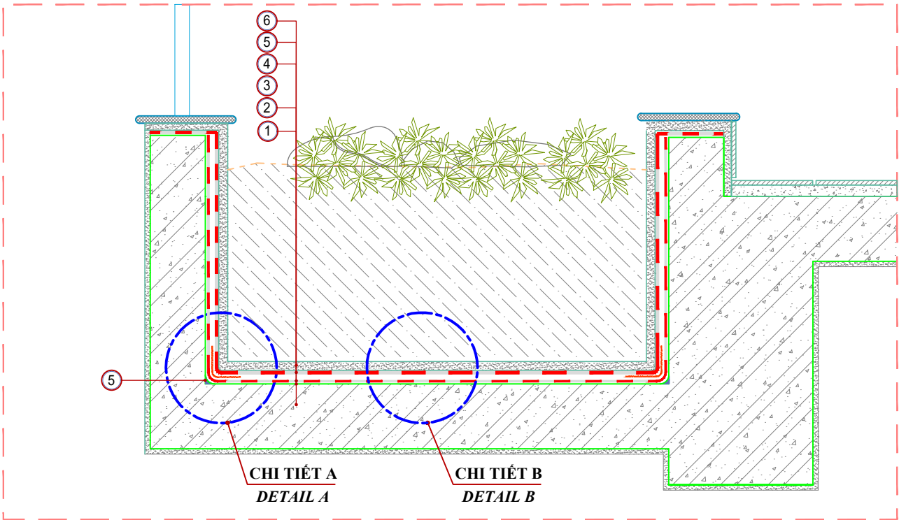
BIỆN PHÁP THI CÔNG CHỐNG THẤM BÒN HOA WATERPROOFING METHOD STATEMENT FOR PLANTER BOX
