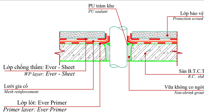
CHI TIẾT XỬ LÝ CỐ ỐNG PIPE TREATMENT
