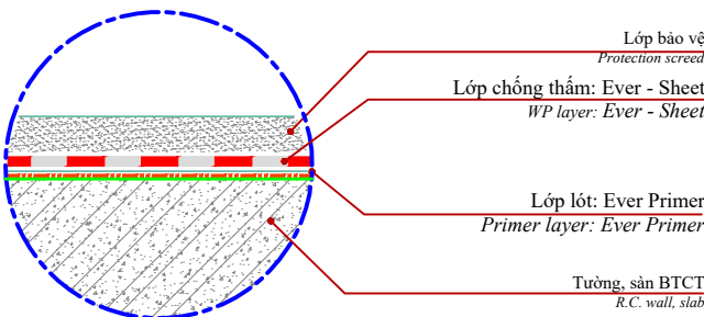
CHI TIẾT B DETAIL B
